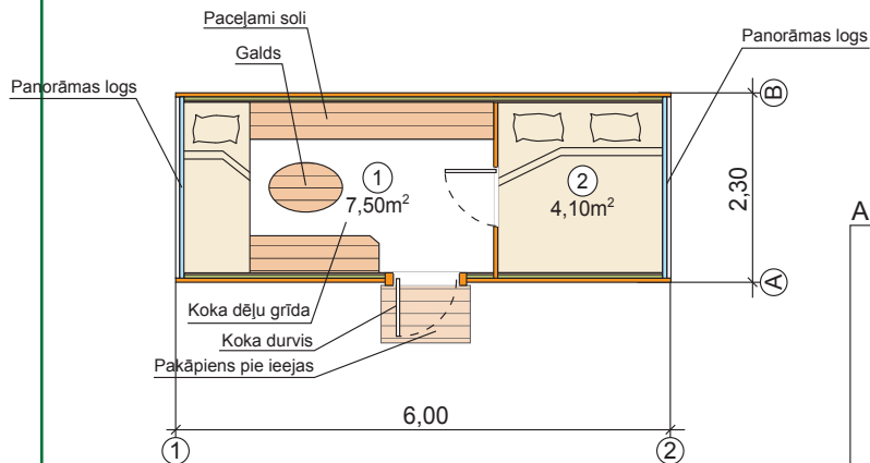
Plāns
