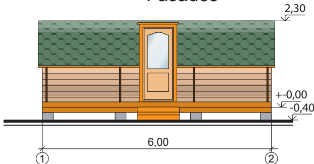
Fasādes
